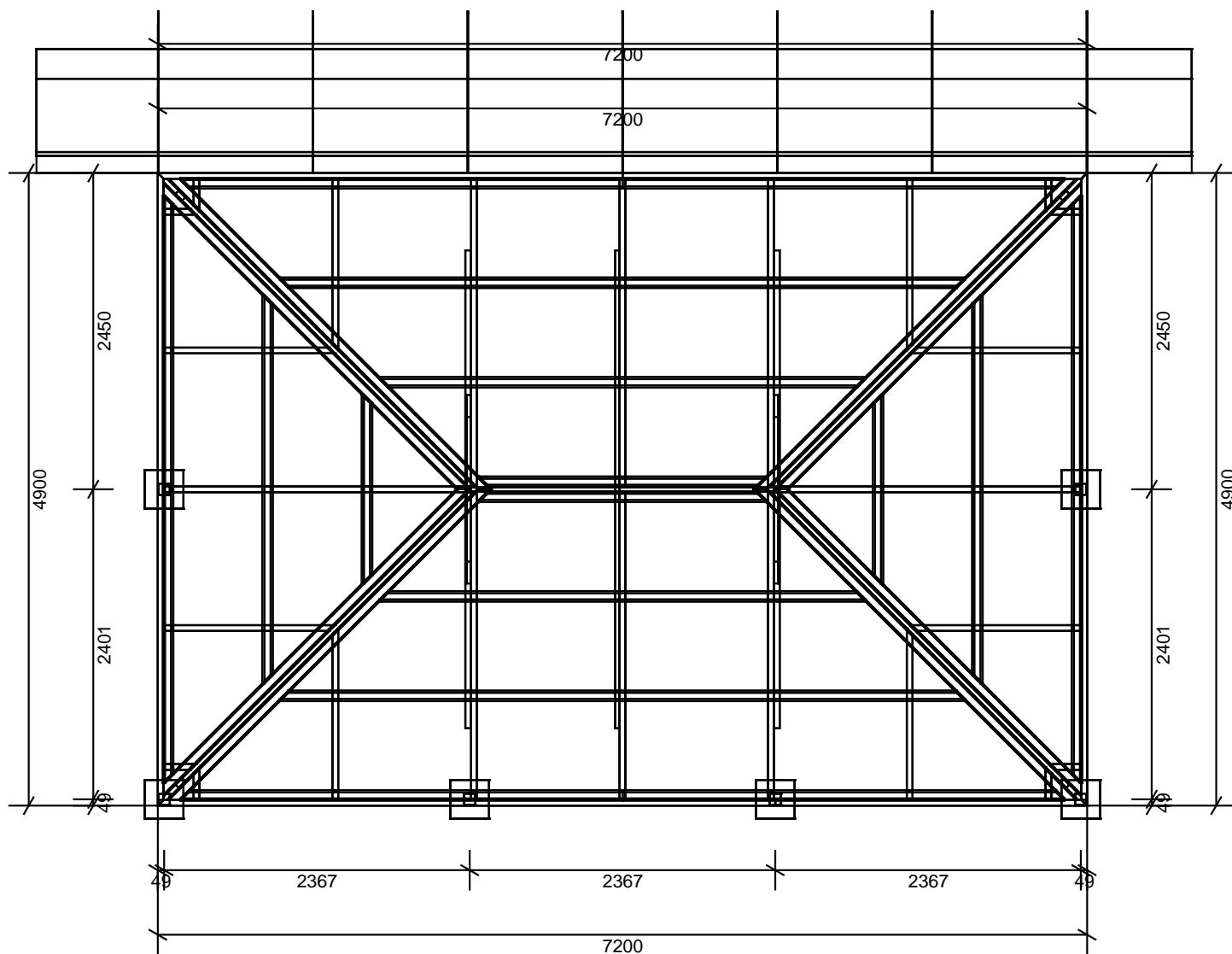
PLAN 1:50
